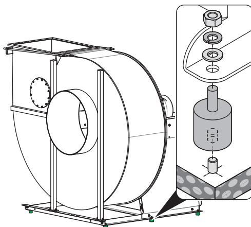
Fig. 27: Proposition de fixation pour montage au sol
