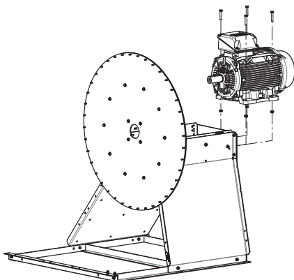
Fig. 38: Démontez le moteur électrique
