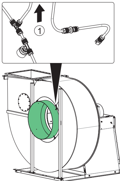
Fig. 17: Point de mesure du débit volumique
