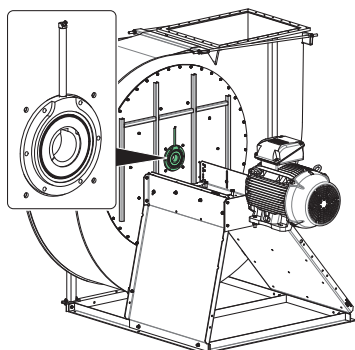
Fig. 11: Joint double avec raccord de regraissage
