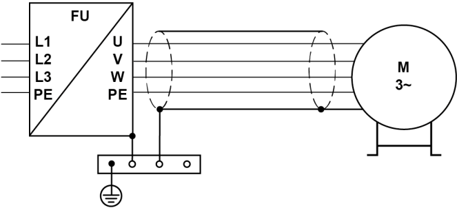
Fig. 32: Principe de raccordement pour le câble court du moteur (CF proche du ventilateur)
