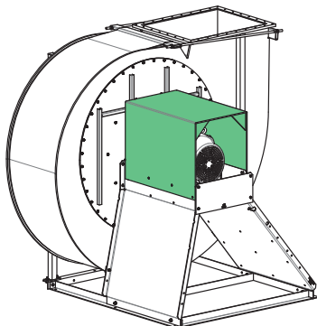
Fig. 9: Capot du moteur
