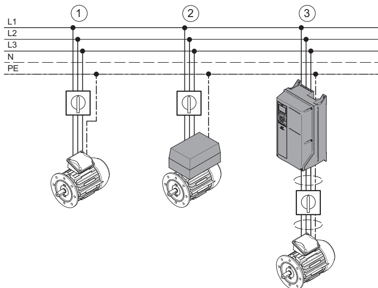
Fig. 31: Options de montage du convertisseur de fréquence
