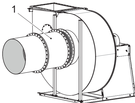
Fig. 28: Raccorder la tuyauterie à la manchette d'aspiration
