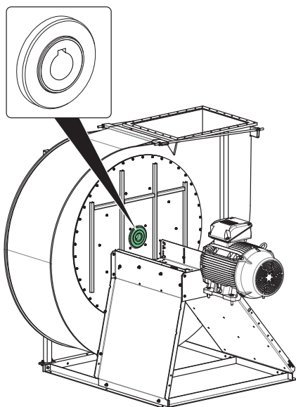
Fig. 14: Anneau de feutre étanchéité du moyeu
