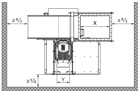
Fig. 24: Besoin de place pour zone de travail et refroidissement du moteur
