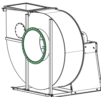
Fig. 6: Raccordement par bride ronde
