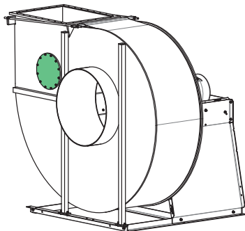
Fig. 26: Montage correct de l'ouverture de contrôle
