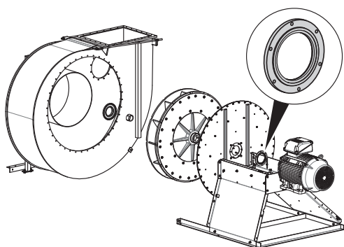
Fig. 39: Remplacer le joint à lèvres
