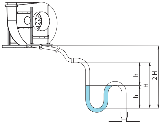
Fig. 30: Hauteur d'installation et de siphon requise
