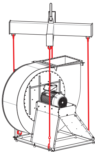
Fig. 22: Ventilateur sur traverse
