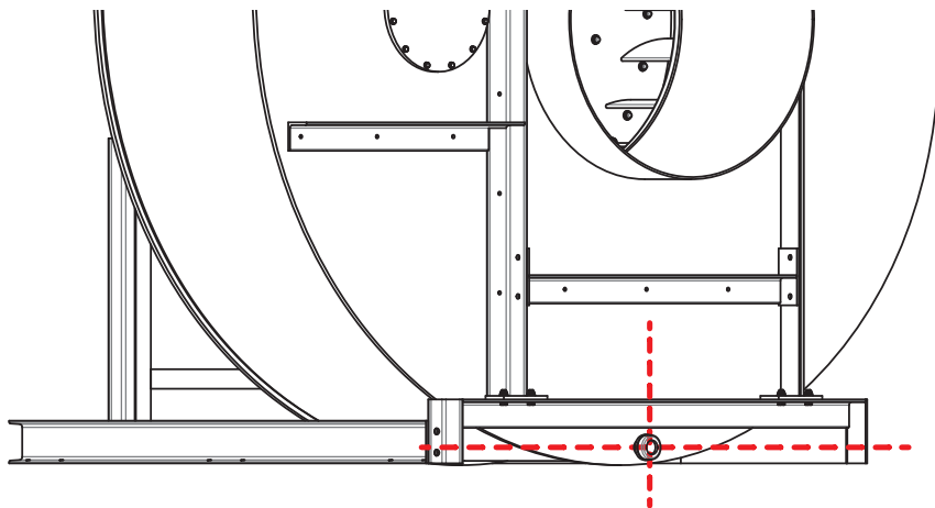
Fig. 29: Position correcte de l'écoulement de condensat
