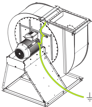
Fig. 34: Prise de terre sur le ventilateur
