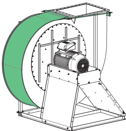
Fig. 25: Montage correct du pare-éclats
