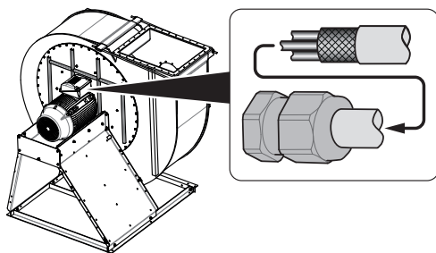
Fig. 33: Presse-étoupe CEM
