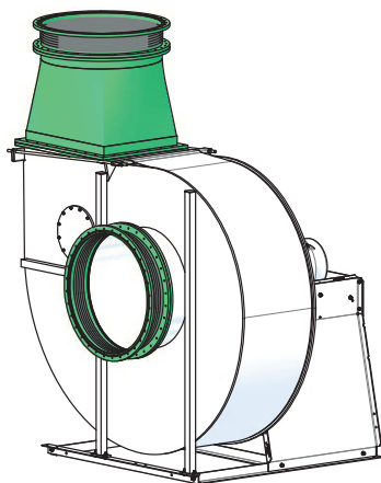
Fig. 5: Manchettes avec bride ronde
