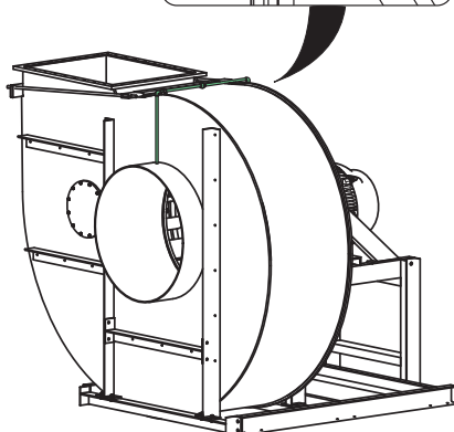
Fig. 12: Réaspiration
