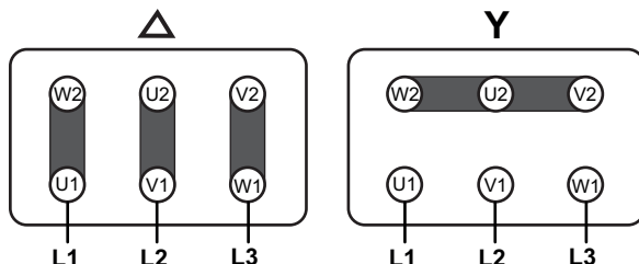
Fig. 35: Affectation des broches pour le montage étoile ou triangle
