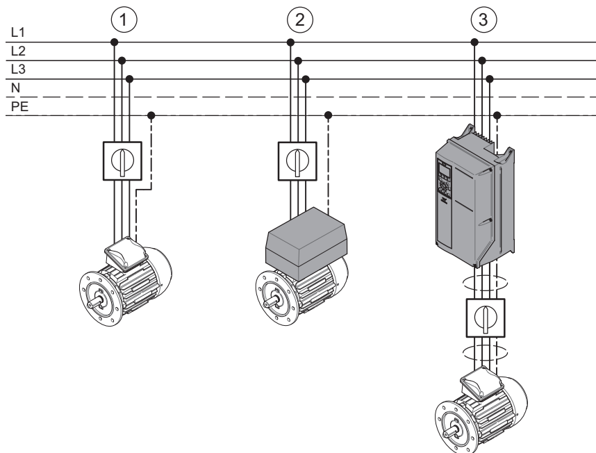
Fig. 31: Options de montage du convertisseur de fréquence
