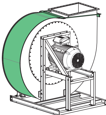
Fig. 25: Montage correct du pare-éclats
