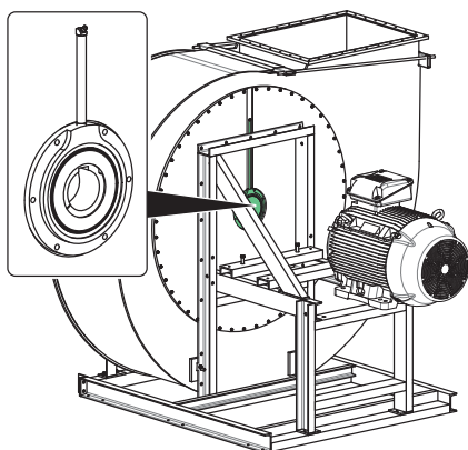
Fig. 11: Joint double avec raccord de graissage
