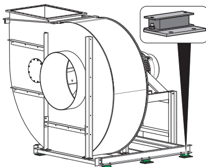
Fig. 4: Amortisseur de vibrations pour montage au sol
