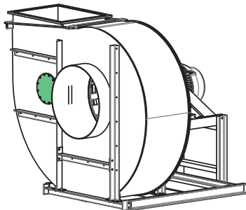
Fig. 26: Montage correct de l'ouverture de contrôle
