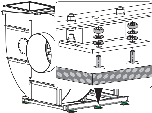
Fig. 27: Proposition de fixation pour montage au sol
