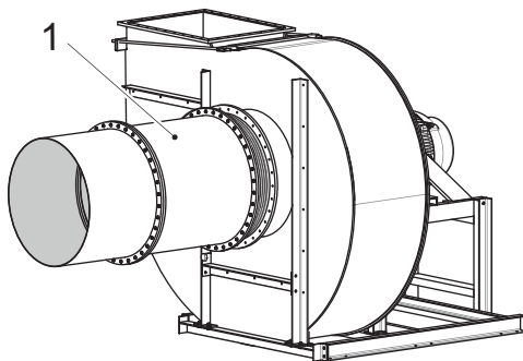
Fig. 28: Raccorder la tuyauterie à la manchette d'aspiration
