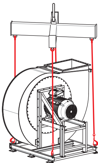
Fig. 22: Ventilateur sur traverse
