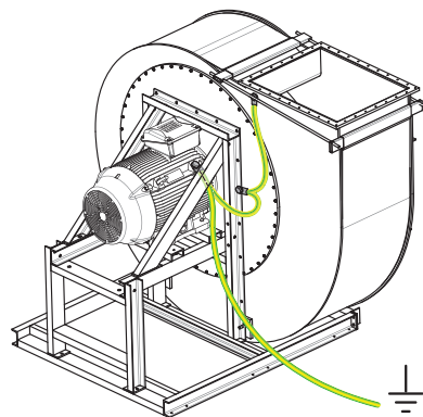
Fig. 34: Prise de terre sur le ventilateur
