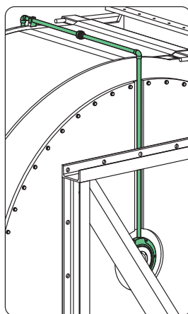
Fig. 11: Joint double avec raccord de graissage
