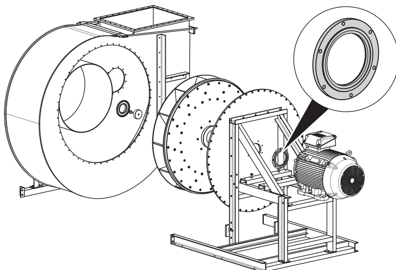
Fig. 39: Remplacer le joint à lèvres
