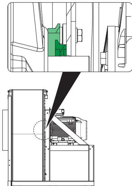
Fig. 15: Etanchéité de moyeu labyrinthe
