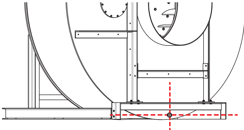
Fig. 29: Position correcte de l'écoulement de condensat
