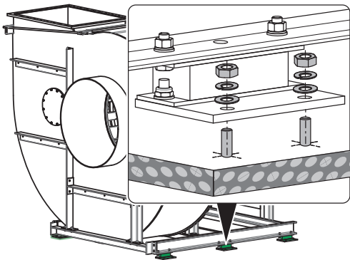
Fig. 28: Proposition de fixation pour montage au sol
