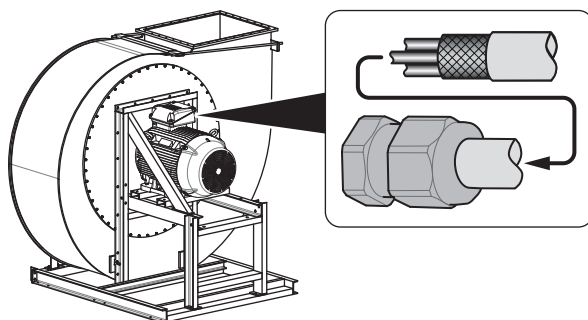
Fig. 34: Presse-étoupe CEM
