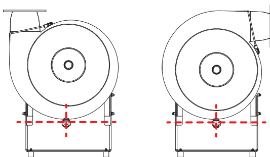
Fig. 27: Position correcte de l'écoulement de condensat
