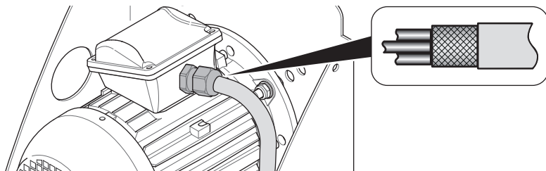
Fig. 30: Presse-étoupe CEM
