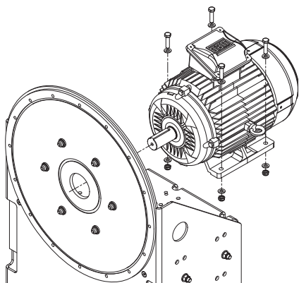
Fig. 35: Démontez le moteur électrique
