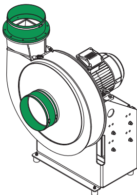
Fig. 5: Positions de montage des manchettes souples
