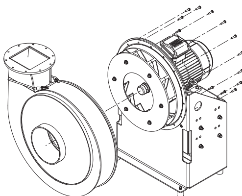
Fig. 32: Démontez la volute
