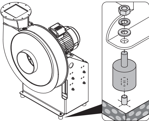
Fig. 25: Proposition de fixation pour montage au sol
