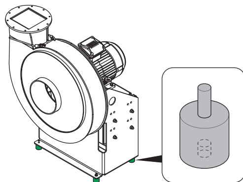
Fig. 4: Amortisseur de vibrations pour montage au sol
