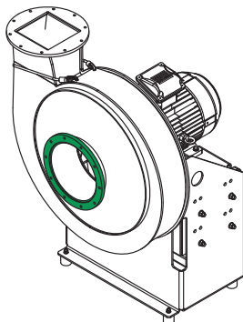
Fig. 7: Raccordements par bride
