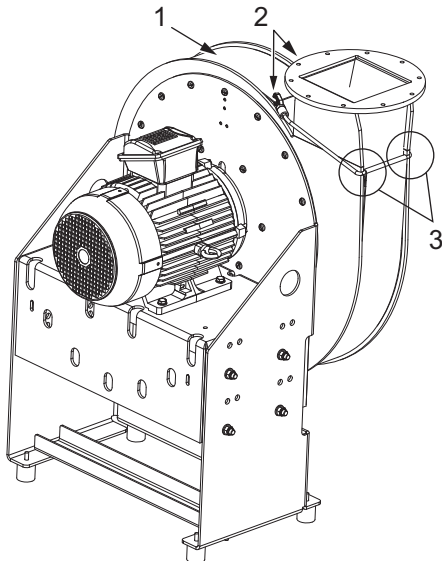
Fig. 24: Montage correct du pare-éclats
