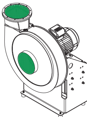
Fig. 12: Grille de protection
