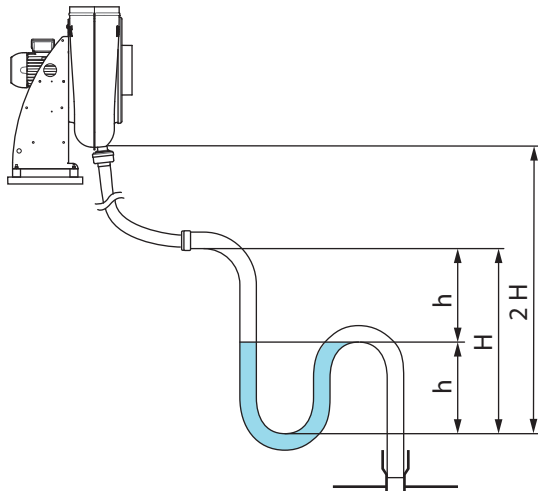
Fig. 28: Hauteur d'installation et de siphon requise
