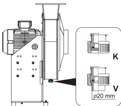
Fig. 8: Écoulement de condensat sur l'évacuation du condensat
