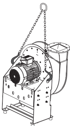
Fig. 21: Ventilateur avec chaîne de levage
