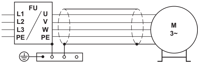
Fig. 29: Principe de raccordement pour le câble court du moteur (CF proche du ventilateur)
