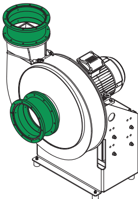
Fig. 6: Manchettes avec bride
