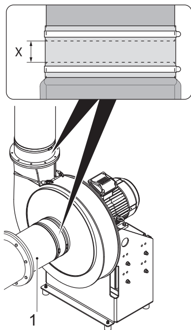
Fig. 26: Plage de distance des raccordements de tuyau
