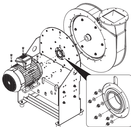
Fig. 36: Remplacez le joint à lèvre
