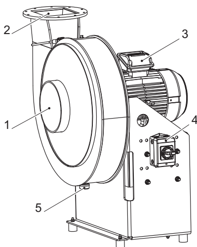
Fig. 1: Interfaces sur le ventilateur
