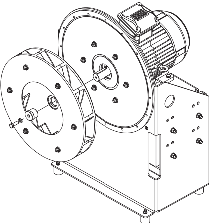
Fig. 34: Démontez la roue du ventilateur
