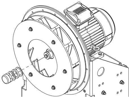
Fig. 33: Retirer le raccord de moyeu.
