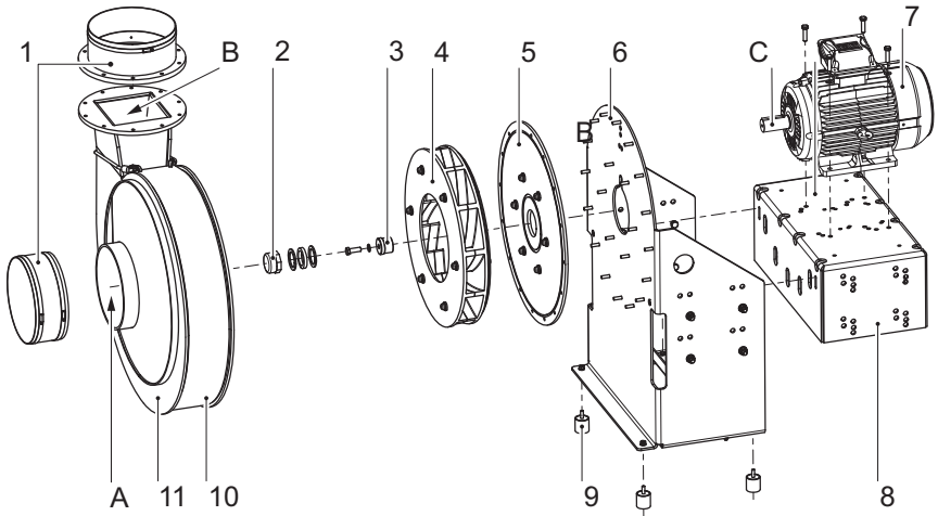
Fig. 2: Vue d'ensemble du ventilateur
