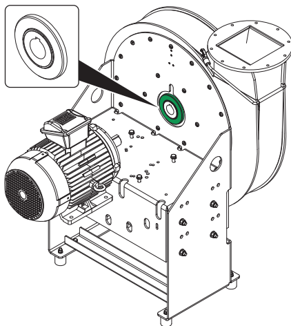
Fig. 17: Anneau de feutre étanchéité du moyeu
