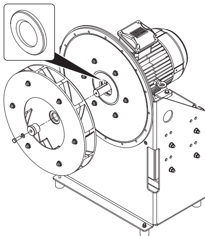
Fig. 37: Remplacer l'étanchéité du moyeu du joint annulaire en feutre
