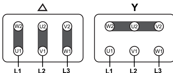
Fig. 31: Affectation des broches pour la commutation étoile ou triangle
