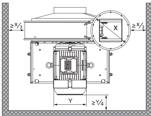
Fig. 23: Besoin de place pour zone de travail et refroidissement du moteur
