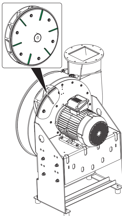
Fig. 18: Roue ailettes dorsales
