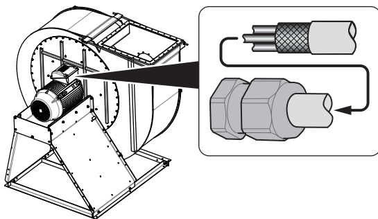
Fig. 33: Presse-étoupe CEM
