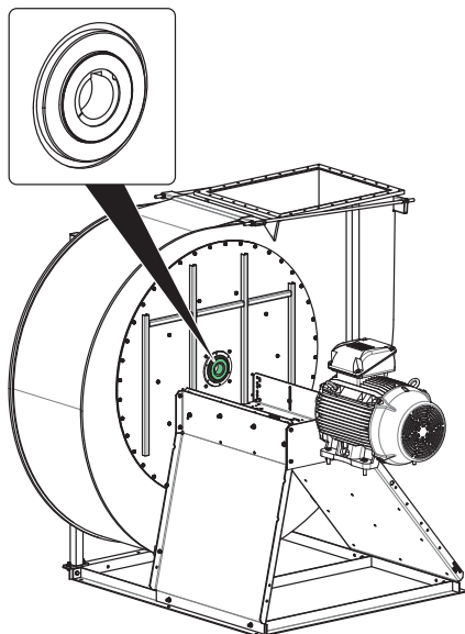
Fig. 10: Joint d'étanchéité à lèvres (simple)
