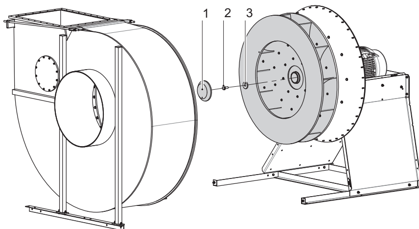
Fig. 37: Remplacement de la roue du ventilateur
