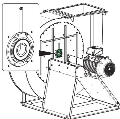
Fig. 11: Joint double avec raccord de graissage
