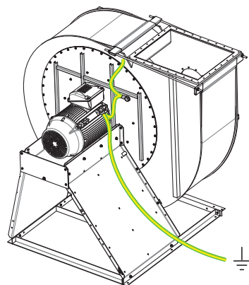
Fig. 34: Prise de terre sur le ventilateur
