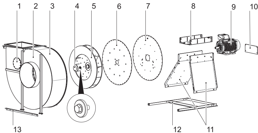
Fig. 2: Vue d'ensemble du ventilateur
