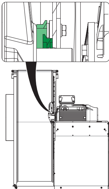
Fig. 15: Etanchéité de moyeu labyrinthe
