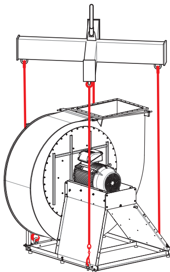
Fig. 22: Ventilateur sur traverse
