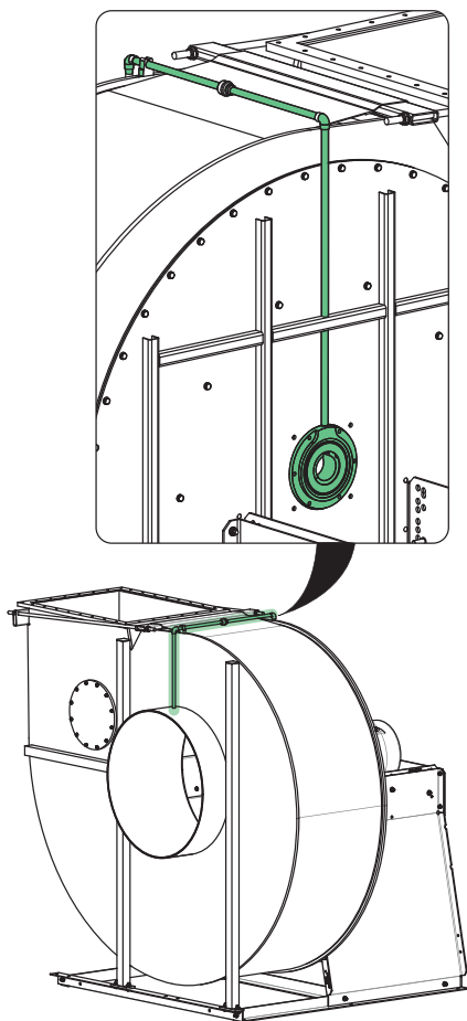
Fig. 12: Réaspiration
