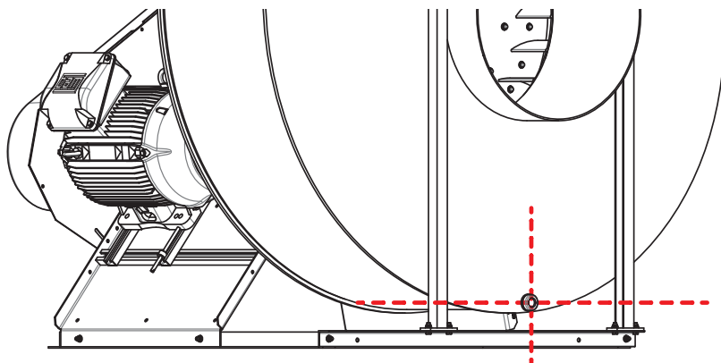
Fig. 30: Position correcte de l'écoulement de condensat
