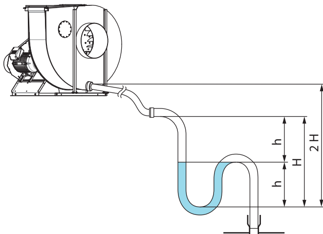
Fig. 31: Hauteur d'installation et de siphon requise
