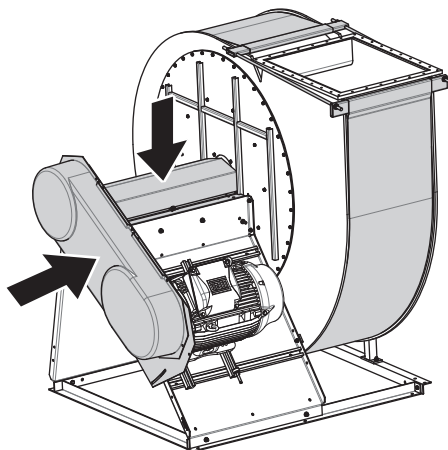
Fig. 32: Contrôler le pare-éclats et les couvercles de protection
