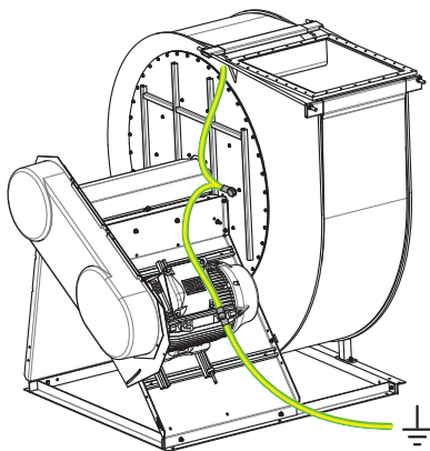
Fig. 36: Prise de terre sur le ventilateur
