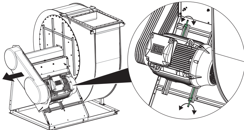
Fig. 26: Contrôler l'entraînement par courroie
