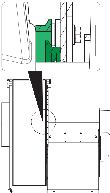
Fig. 15: Etanchéité de moyeu labyrinthe
