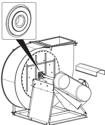
Fig. 14: Anneau de feutre étanchéité du moyeu
