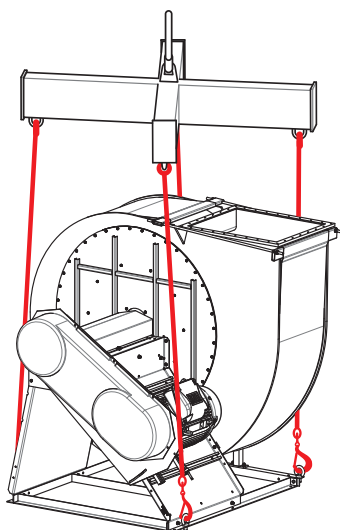
Fig. 22: Ventilateur sur traverse
