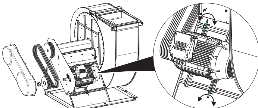
Fig. 45: Remplacez la courroie d'entraînement
