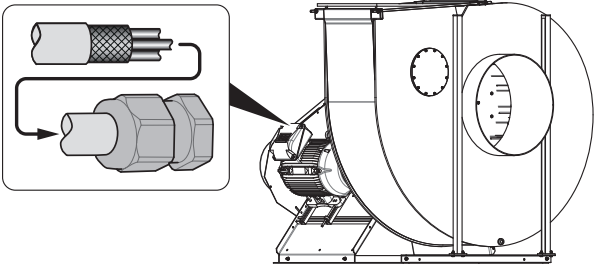
Fig. 35: Presse-étoupe CEM
