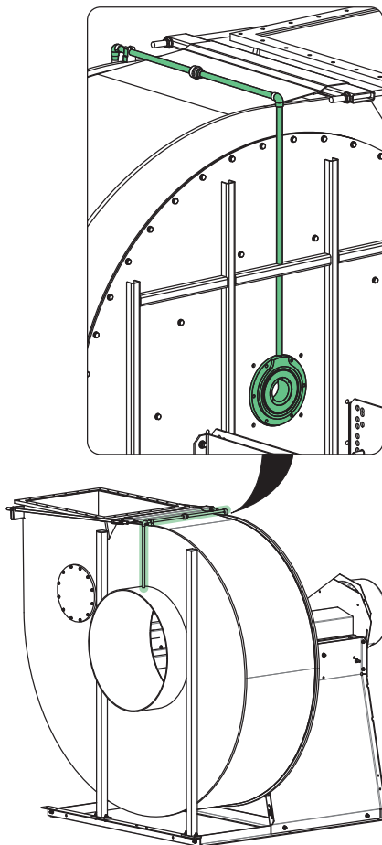
Fig. 12: Réaspiration
