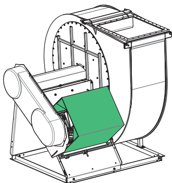
Fig. 9: Capot du moteur
