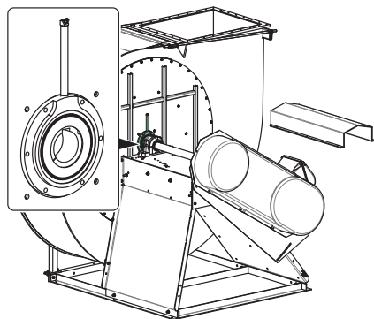
Fig. 11: Joint double avec raccord de graissage
