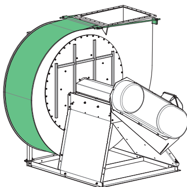
Fig. 25: Montage correct du pare-éclats
