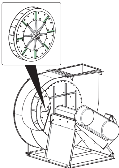
Fig. 16: Roue ailettes dorsales
