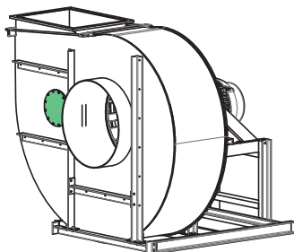
Fig. 26: Montage correct de l'ouverture de contrôle
