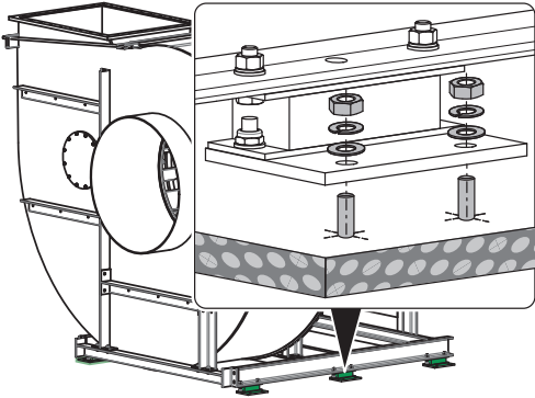
Fig. 27: Proposition de fixation pour montage au sol
