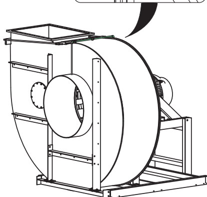
Fig. 12: Réaspiration
