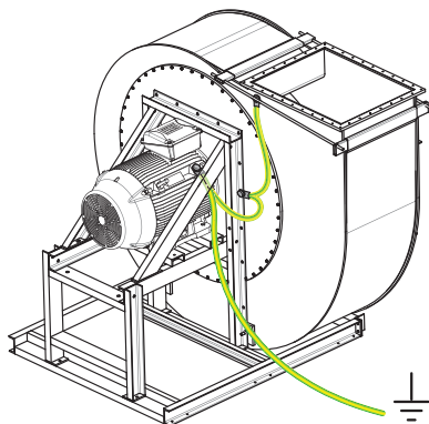
Fig. 34: Prise de terre sur le ventilateur
