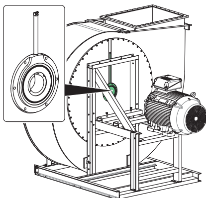
Fig. 11: Joint double avec raccord de regraissage
