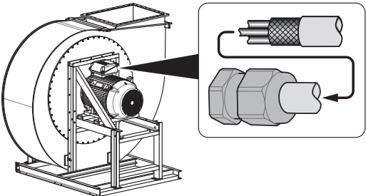
Fig. 33: Presse-étoupe CEM
