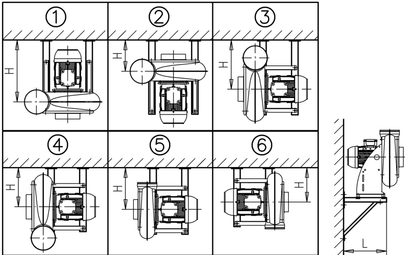
Fig. 27: Position de montage sur la console murale
