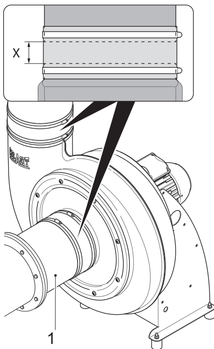
Fig. 29: Plage de distance des raccordements de tuyau
