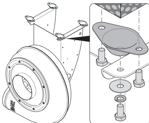
Fig. 28: Proposition de fixation pour montage au plafond
