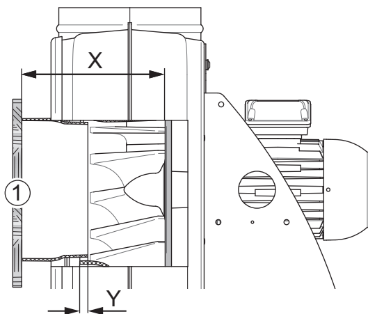
Fig. 42: Mesure la position de la roue du ventilateur (vue en coupe)
