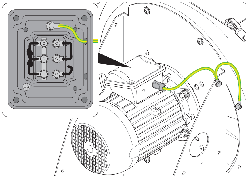
Fig. 34: Câble de mise à la terre sur le ventilateur
