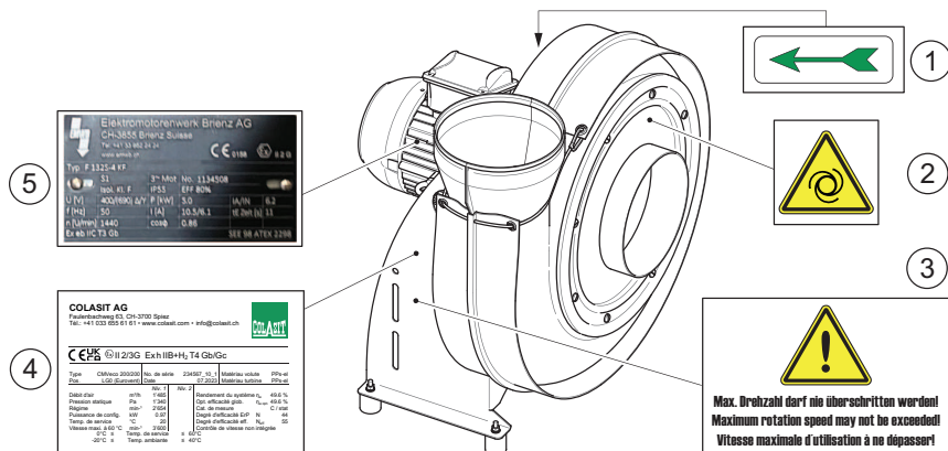
Fig. 3: Plaques et symboles d'avertissement sur le ventilateur
