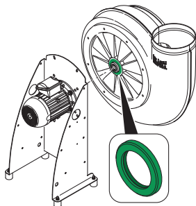
Fig. 17: Anneau de feutre étanchéité du moyeu
