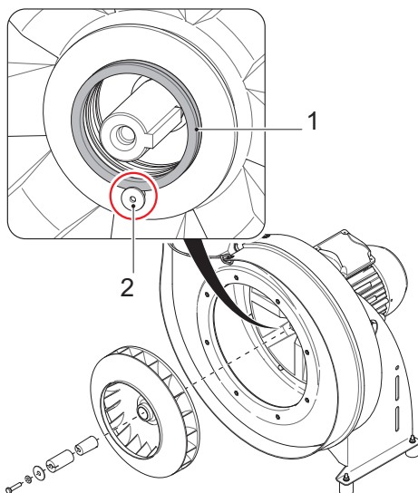
Fig. 43: Remplacez le joint V-ring
