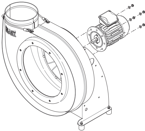
Fig. 41: Démontez le moteur électrique (ED)
