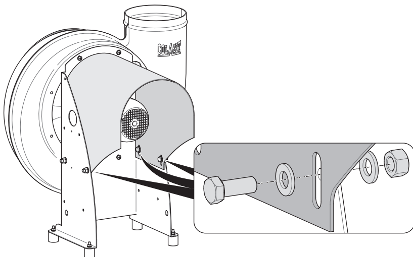
Fig. 36: Monter le capot du moteur (ED)
