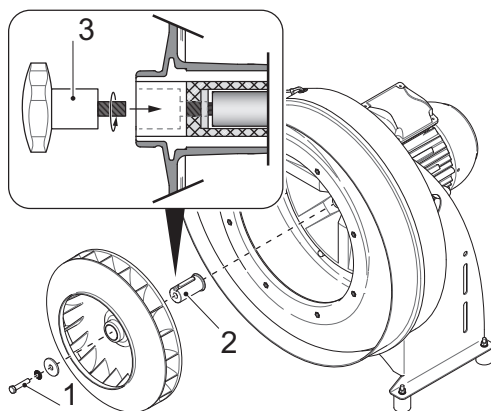
Fig. 39: Démontez la roue du ventilateur
