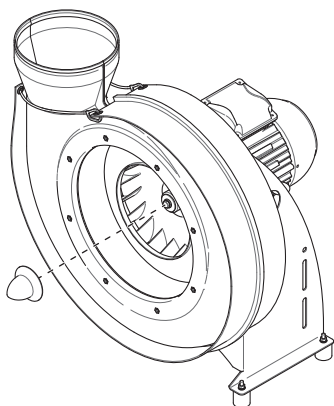
Fig. 38: Retirez le capuchon du moyeu
