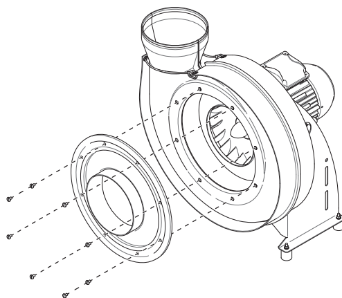
Fig. 37: Démontez le couvercle d'admission
