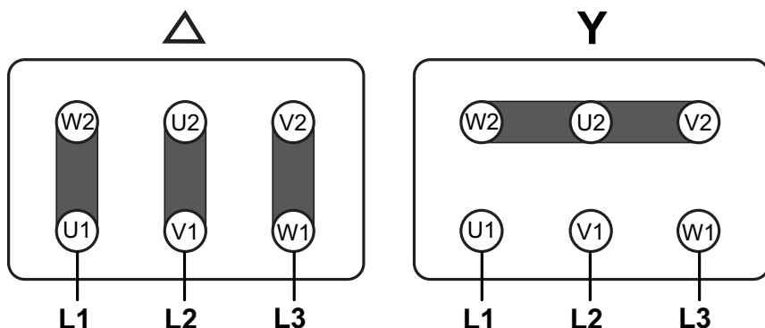
Fig. 35: Affectation des broches pour la commutation triangle et étoile
