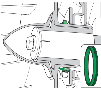
Fig. 16: Étanchéité du moyeu V-Ring
