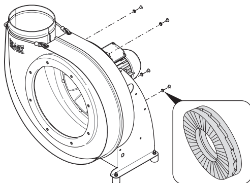
Fig. 40: Démontez la volute
