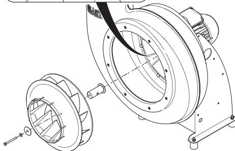
Fig. 44: Remplacez l'étanchéité du moyeu de l'anneau de feutre
