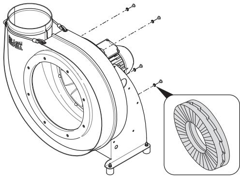
Fig. 39: Démontez la volute
