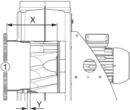
Fig. 41: Mesurez la position de la roue du ventilateur (vue en coupe)
