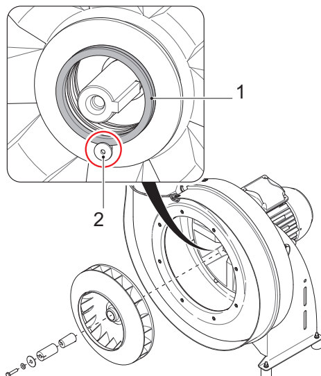
Fig. 42: Remplacez le joint V-ring
