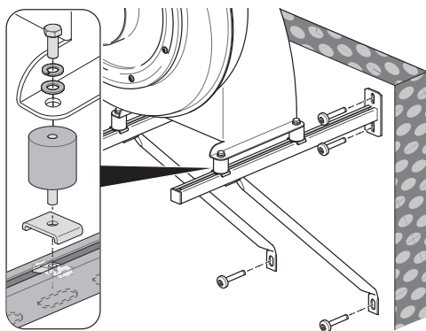
Fig. 26: Proposition de fixation pour montage mural
