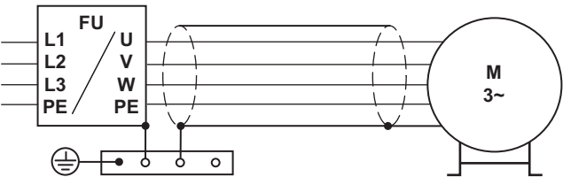
Fig. 32: Principe de raccordement pour le câble court du moteur (CF proche du ventilateur)
