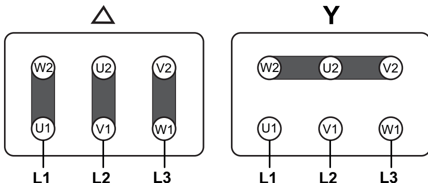
Fig. 34: Affectation des broches pour la commutation triangle et étoile
