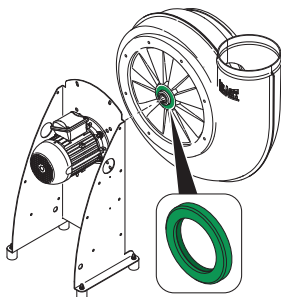
Fig. 17: Anneau de feutre étanchéité du moyeu
