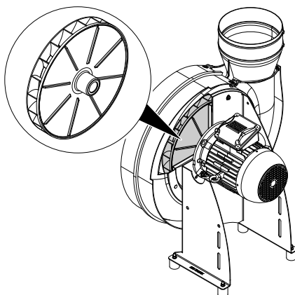
Fig. 18: Roue ailettes dorsales
