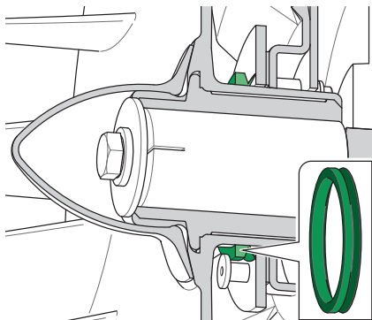
Fig. 16: Étanchéité du moyeu V-Ring
