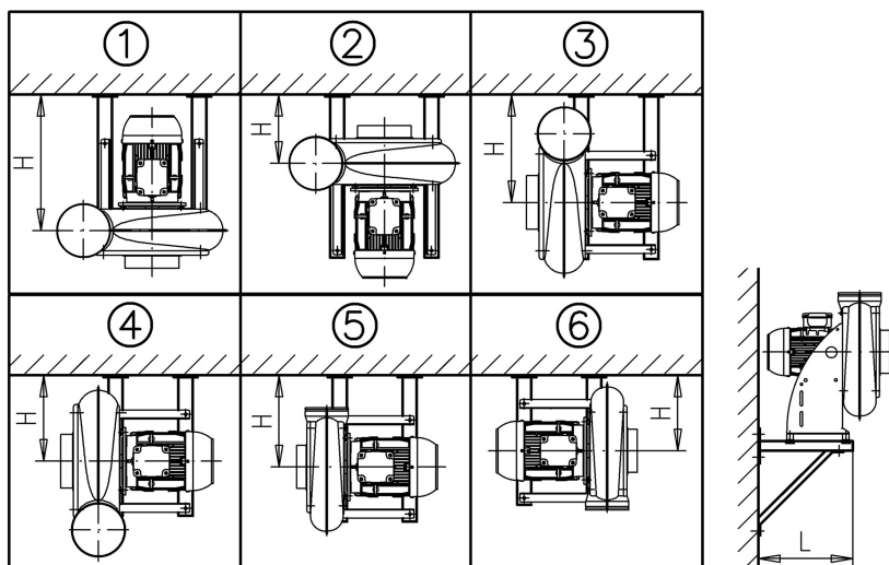
Fig. 27: Position de montage sur la console murale
