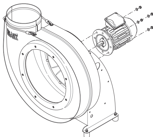
Fig. 40: Démontez le moteur électrique (ED)
