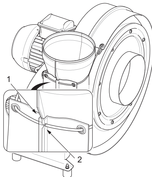
Fig. 24: Montage correct du pare-éclats
