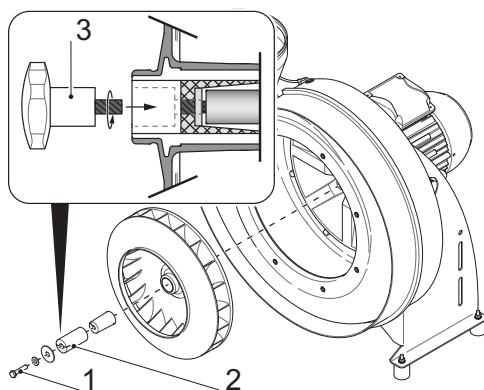
Fig. 38: Démontez la roue du ventilateur
