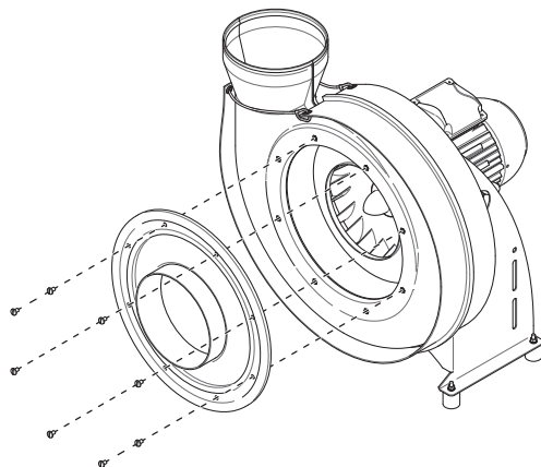
Fig. 36: Démontez le couvercle d'admission
