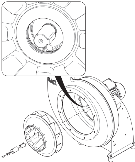
Fig. 43: Remplacez l'étanchéité du moyeu de l'anneau de feutre
