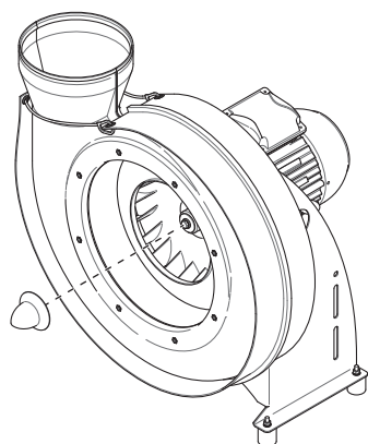
Fig. 37: Retirez le capuchon du moyeu
