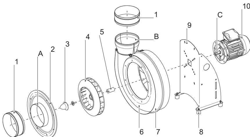
Fig. 2: Vue d'ensemble du ventilateur
