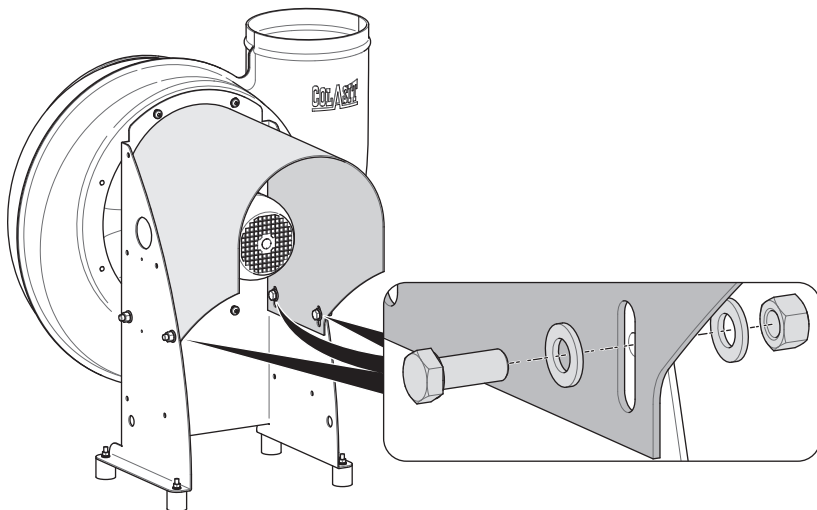
Fig. 35: Monter le capot du moteur (ED)
