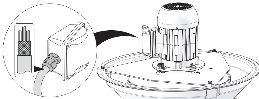
Fig. 16: Presse-étoupe CEM
