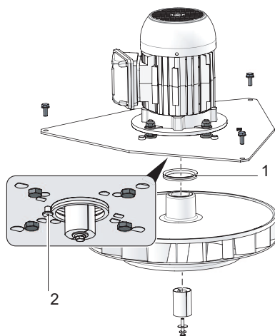
Fig. 23: Remplacer le joint V-Ring
