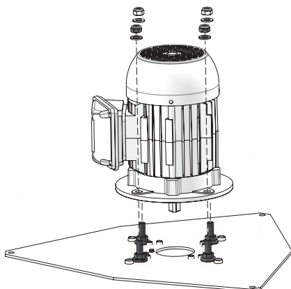
Fig. 21: Démonter le moteur électrique
