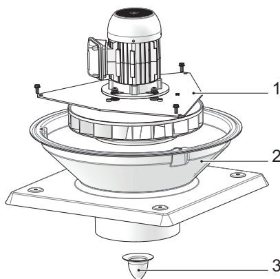
Fig. 19: Retirer le capuchon du moyeu et la plaque de moteur
