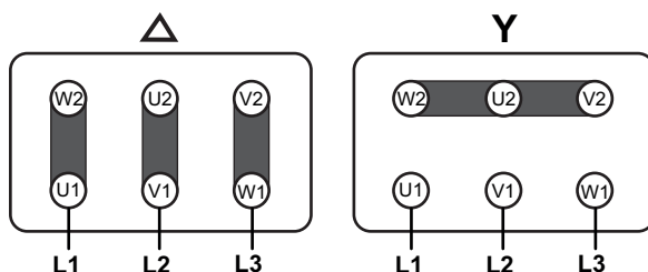
Fig. 17: Affectation des broches pour le montage étoile ou triangle
