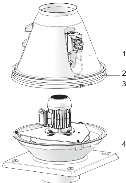
Fig. 18: Démonter la volute
