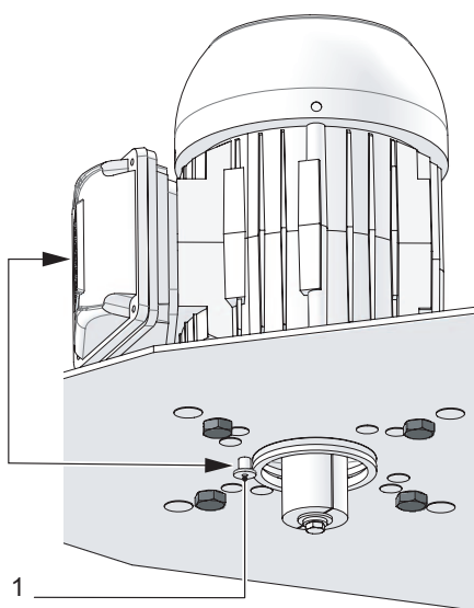
Fig. 22: Positionner le moteur électrique
