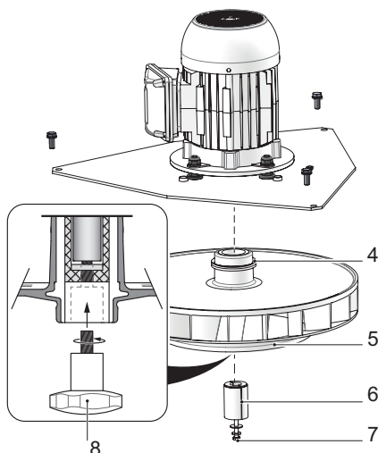
Fig. 20: Démontez la roue du ventilateur
