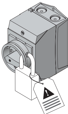
Fig. 4: Interrupteur de révision
