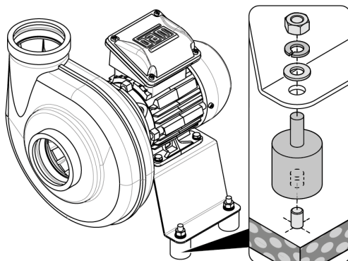
Fig. 12: Proposition de fixation pour montage au sol
