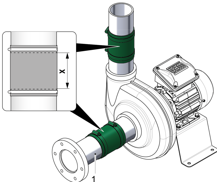
Fig. 13: Plage de distance des raccordements de tuyau
