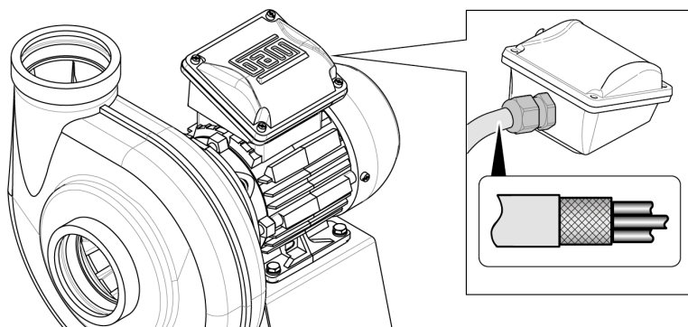
Fig. 16: Presse-étoupe CEM
