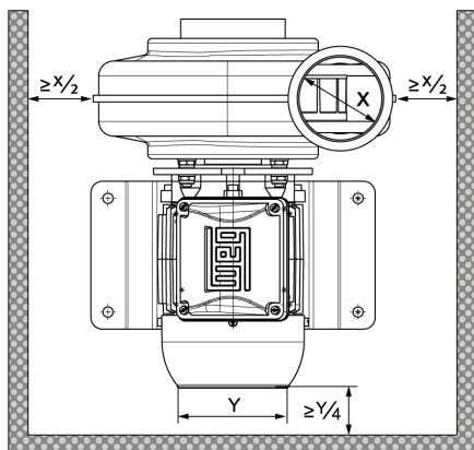
Fig. 11: Besoin de place pour zone de travail et refroidissement du moteur
