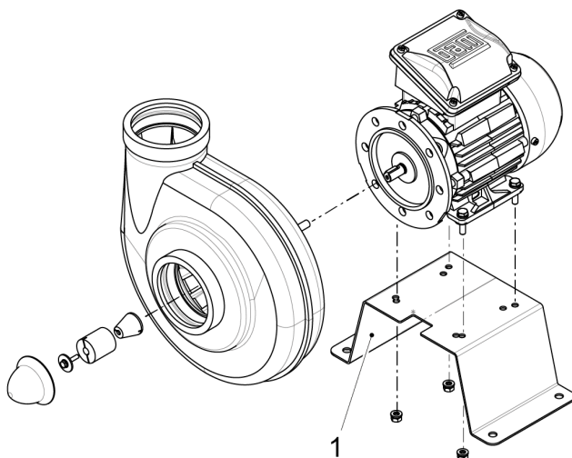
Fig. 19: Démontez le moteur électrique
