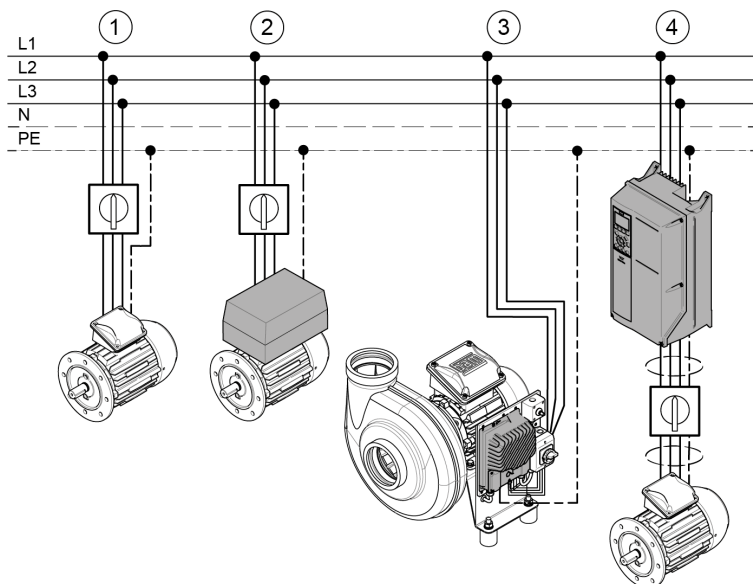
Fig. 14: Options de montage du convertisseur de fréquence (CF)
