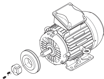
Fig. 37: Démonter le moteur électrique
