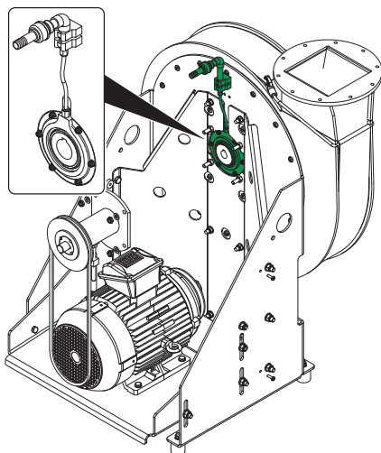
Fig. 16: Gaz d'arrêt
