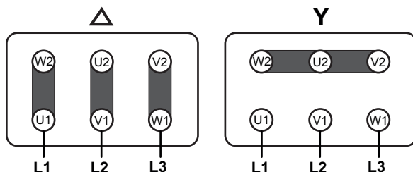
Fig. 32: Affectation des broches pour la commutation étoile ou triangle
