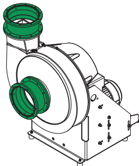
Fig. 6: Manchettes avec bride
