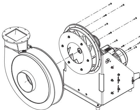
Fig. 34: Démontez la volute
