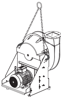
Fig. 21: Ventilateur avec chaîne de levage
