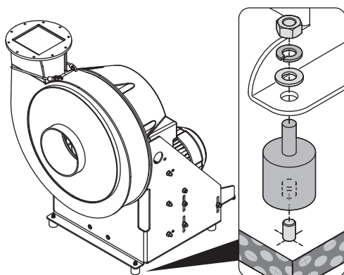
Fig. 26: Proposition de fixation pour montage au sol
