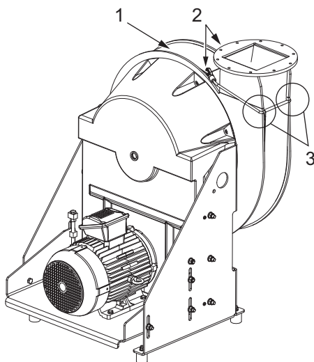
Fig. 25: Montage correct du pare-éclats
