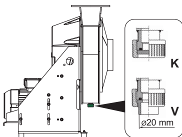
Fig. 8: Écoulement de condensat sur l'évacuation du condensat
