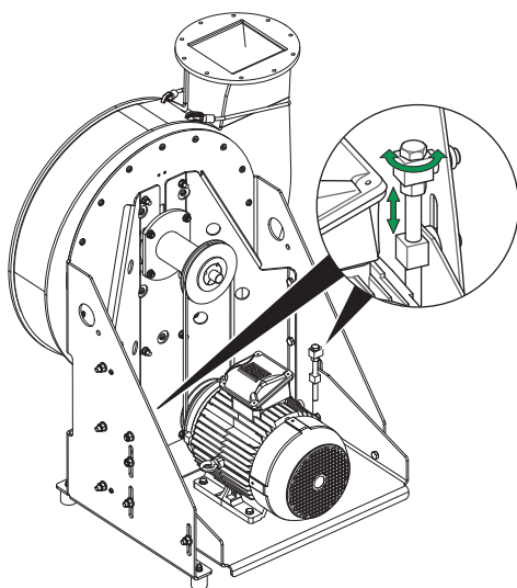
Fig. 24: Contrôler l'entraînement par courroie
