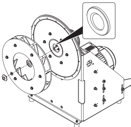
Fig. 40: Remplacer l'étanchéité du moyeu du joint annulaire en feutre
