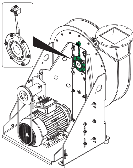
Fig. 14: Joint double avec raccord de graissage
