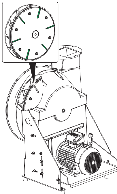
Fig. 18: Roue ailettes dorsales
