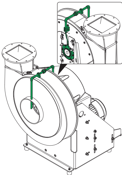
Fig. 15: Réaspiration
