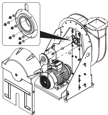
Fig. 39: Remplacer le joint à lèvre
