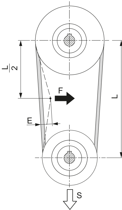
Fig. 42: Mesurez la tension de la courroie
