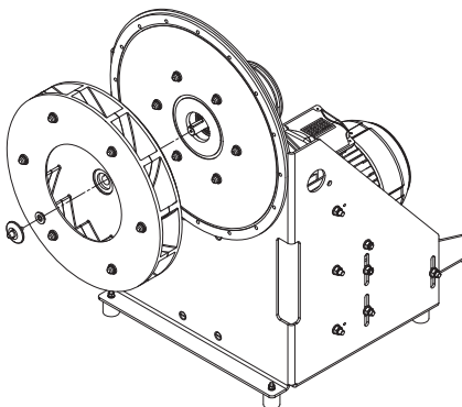
Fig. 36: Démontez la roue du ventilateur
