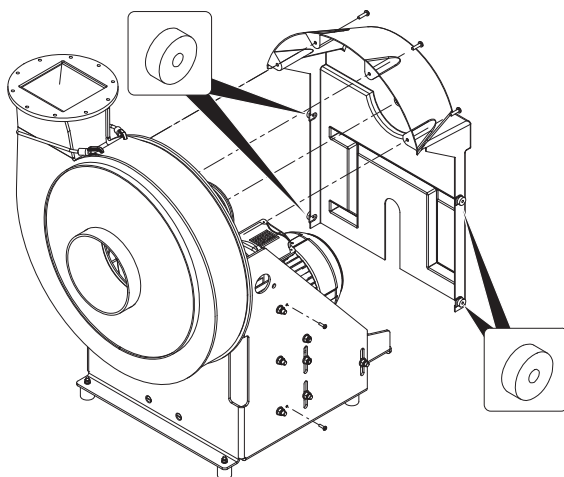
Fig. 33: Monter la protection de la courroie trapézoïdale
