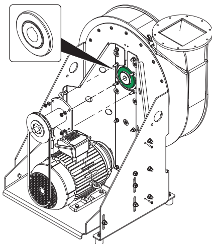
Fig. 17: Anneau de feutre étanchéité du moyeu
