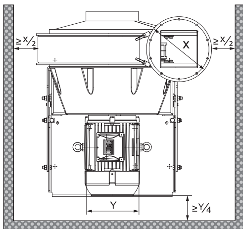
Fig. 23: Besoin de place pour zone de travail et refroidissement du moteur
