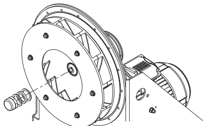
Fig. 35: Retirer le raccord de moyeu.
