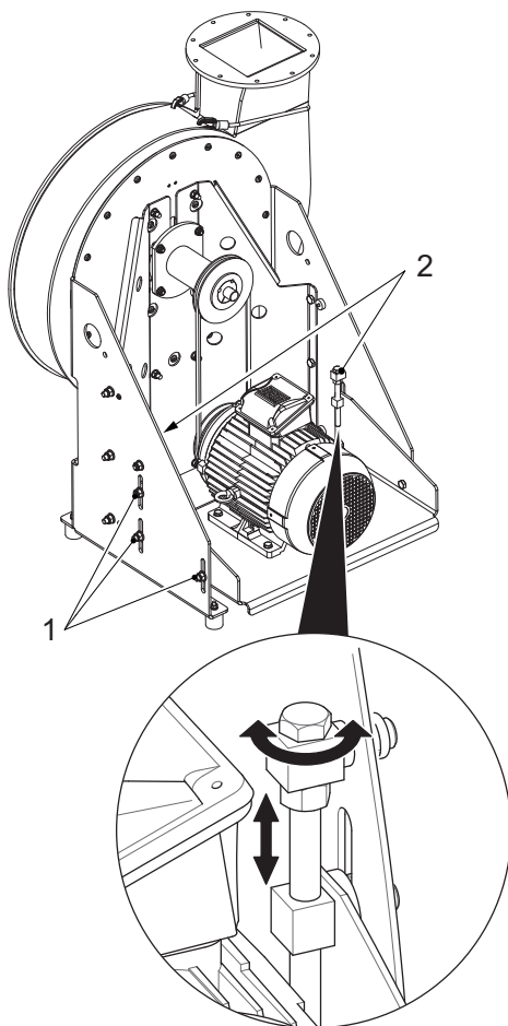
Fig. 41: Remplacez la courroie d'entraînement
