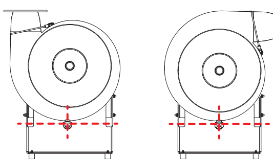
Fig. 28: Position correcte de l'écoulement de condensat
