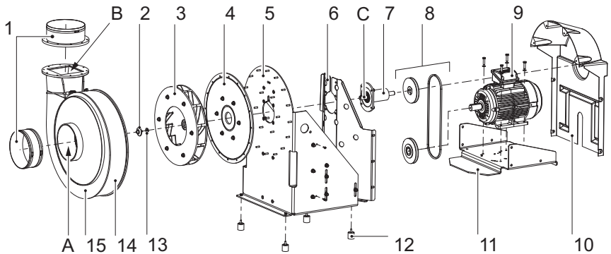
Fig. 2: Vue d'ensemble du ventilateur
