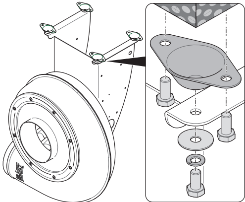
Fig. 27: Proposition de fixation pour montage au plafond
