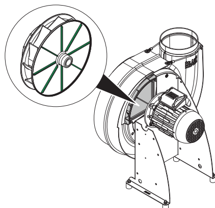
Fig. 17: Roue ailettes dorsales
