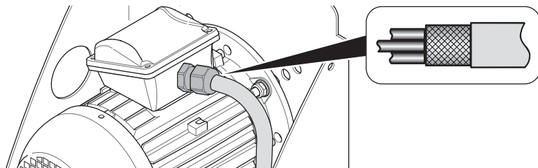
Fig. 32: Presse-étoupe CEM
