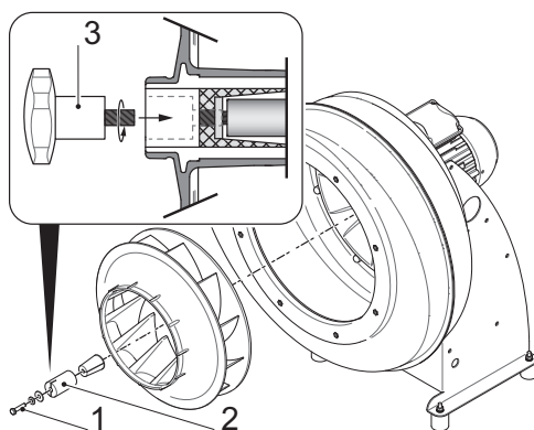
Fig. 37: Démontez la roue du ventilateur
