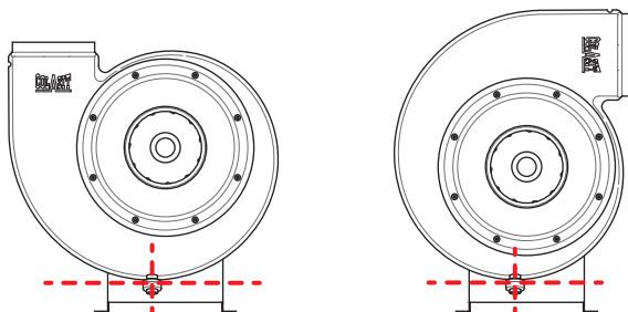
Fig. 29: Position correcte de l'écoulement de condensat
