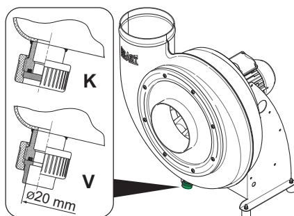
Fig. 9: Écoulement de condensat sur l'évacuation du condensat
