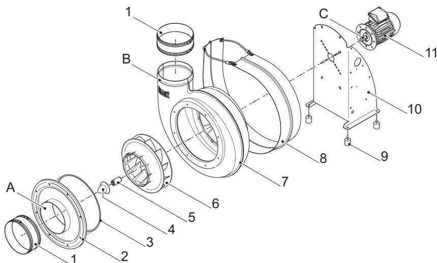
Fig. 2: Vue d'ensemble du ventilateur
