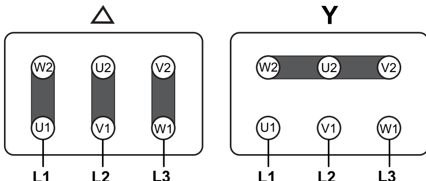
Fig. 33: Affectation des broches pour la commutation triangle et étoile
