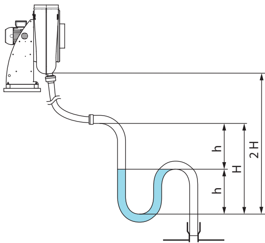
Fig. 30: Hauteur d'installation et de siphon requise
