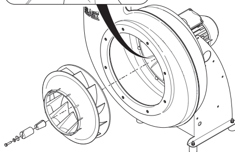
Fig. 40: Remplacez l'étanchéité du moyeu de l'anneau de feutre
