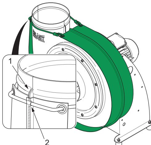
Fig. 23: Montage correct du pare-éclats
