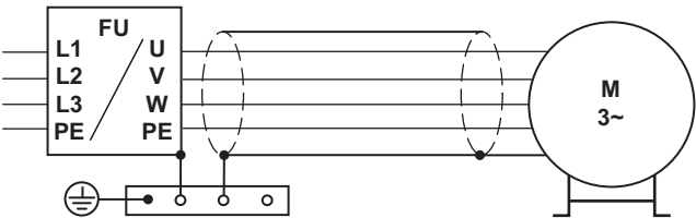
Fig. 31: Principe de raccordement pour le câble court du moteur (CF proche du ventilateur)
