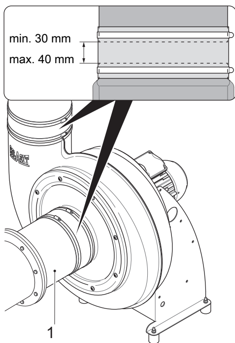
Fig. 28: Plage de distance des raccordements de tuyau
