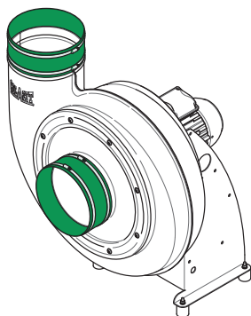
Fig. 6: Positions de montage des manchettes souples
