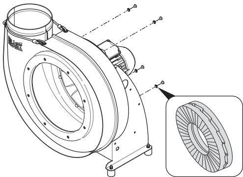
Fig. 38: Démontez la volute
