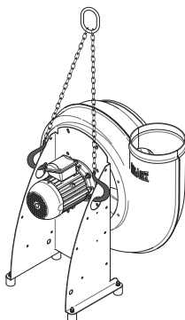
Fig. 20: Ventilateur avec chaîne de levage
