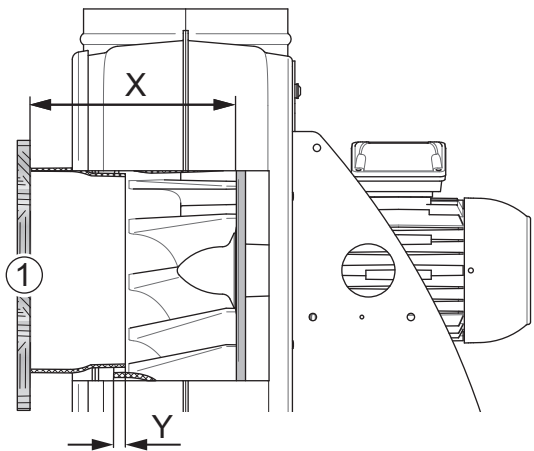
Fig. 39: Mesurez la position de la roue du ventilateur (vue en coupe)
