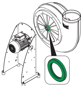
Fig. 16: Anneau de feutre étanchéité du moyeu
