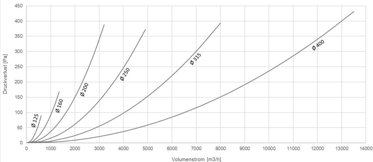
Druckverlust / Volumenstrom
