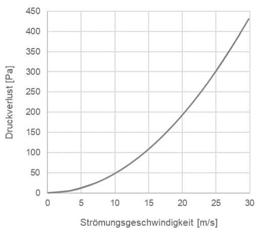
Druckverlust / Strömungsgesch.
